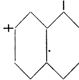
Liebmann u. Studer. Pat.-Anm. 4327 v. 6. Juni 1887.
